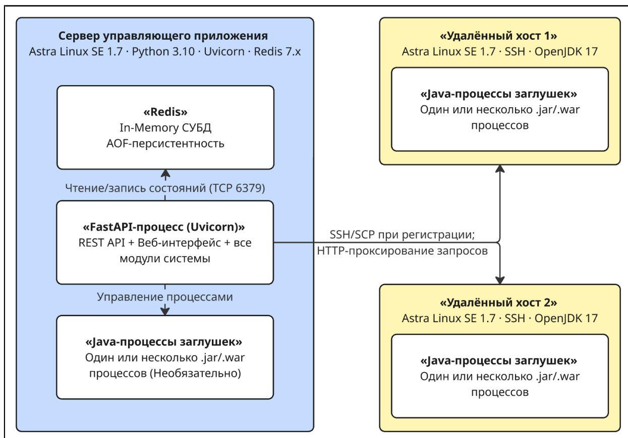
Рисунок 4 – Диаграмма развёртывания
